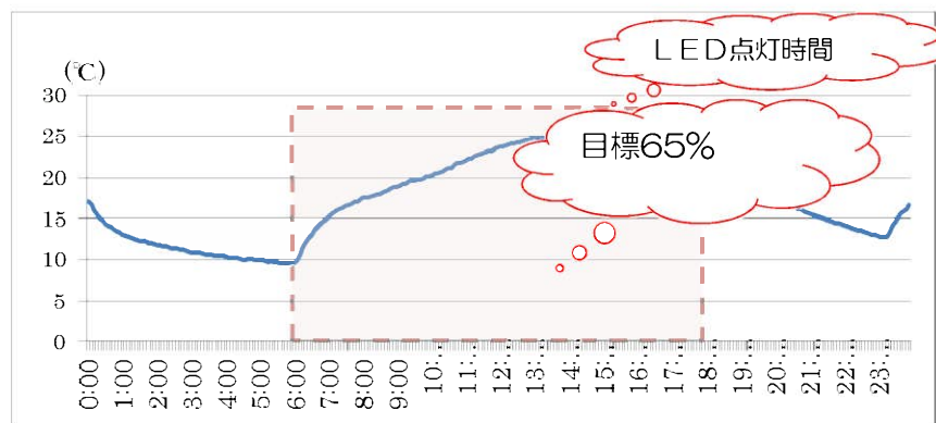
図5. 2 LED点灯時間と室温変化の推移
