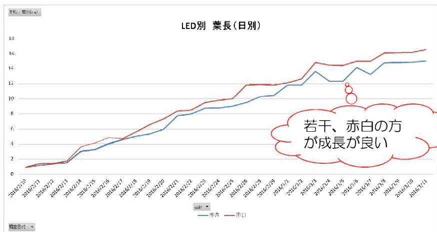
図3.5 レタスのLED波長比較
