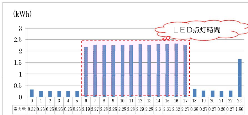
図5. 1 1日の消費電力推移 (ユニットハウス) 外気温と室温のデータ 《2月》
