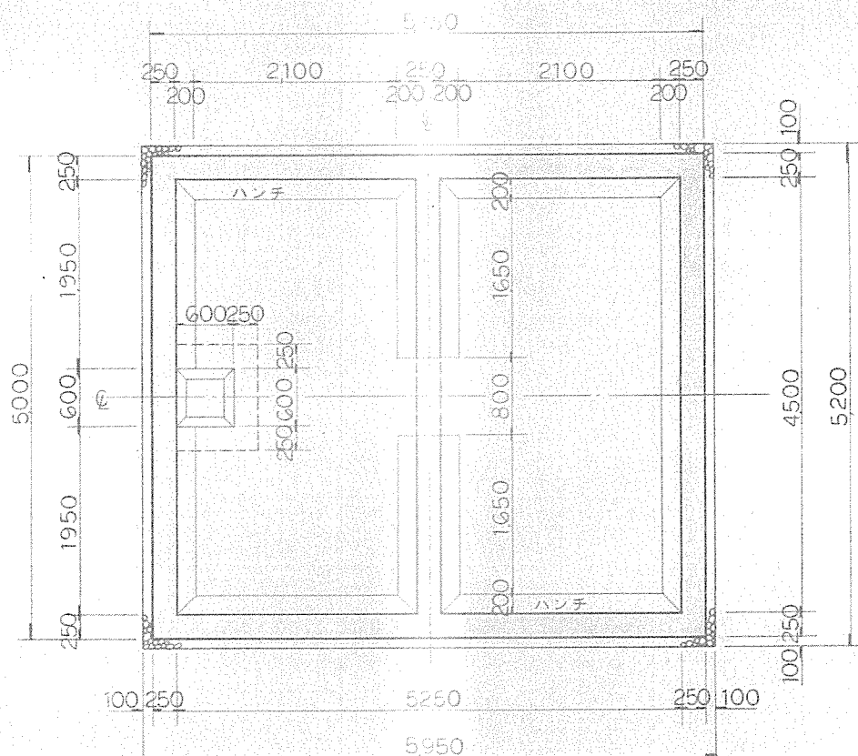
底版平面図 S-1:50
