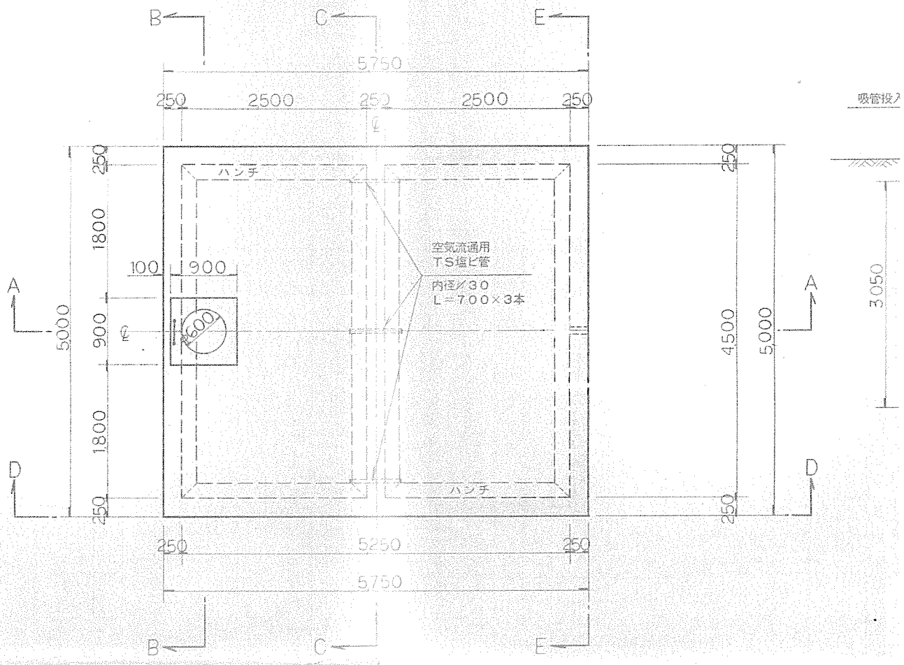
底版平面図 S-1:50
