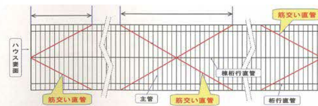
筋交いによる妻面の補強方法事例
